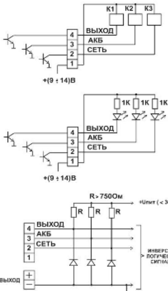
Рисунок 2. Примеры схем подключения исполнительных устройств к выходам «открытый коллектор»
