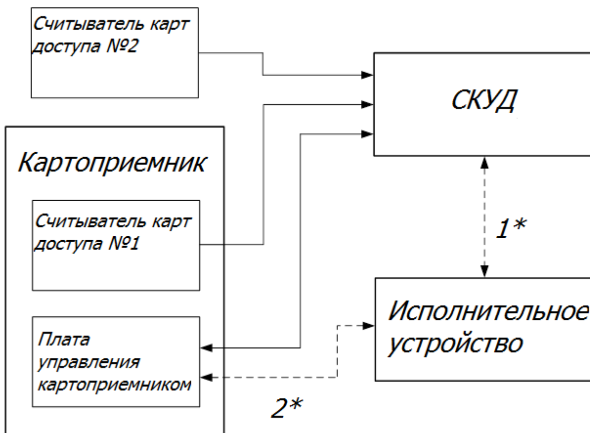
Рисунок 15 – Структурная схема №1
