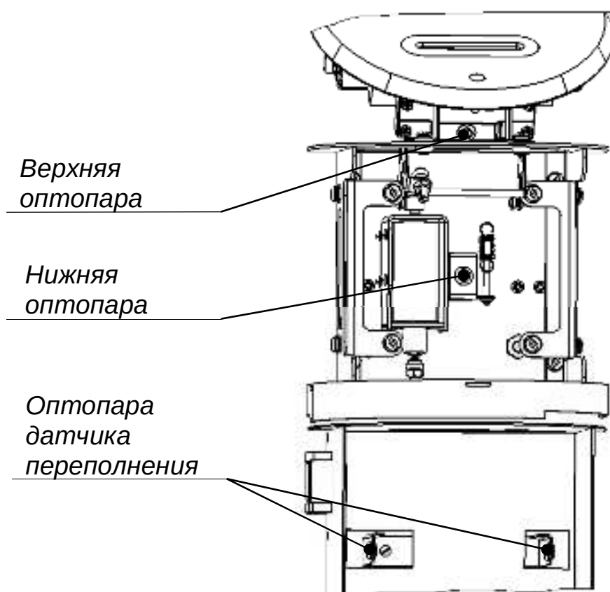
Рис. 7. Расположение оптопар картоприемника
