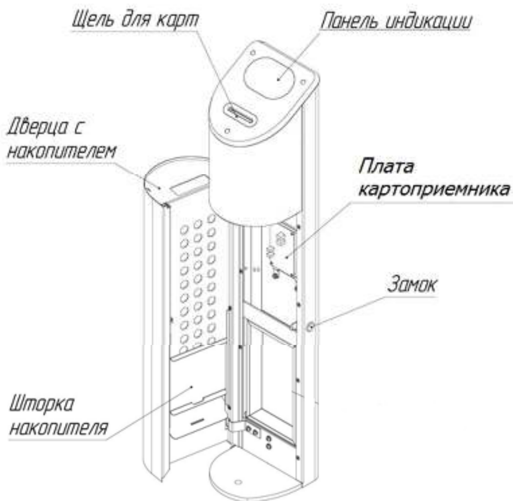
Рис. 5. Общий вид картоприемника
