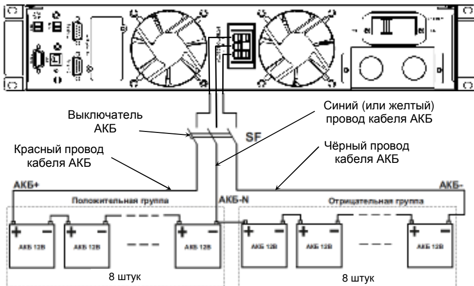
Рисунок 4 — Схема монтажа аккумуляторной батареи.
