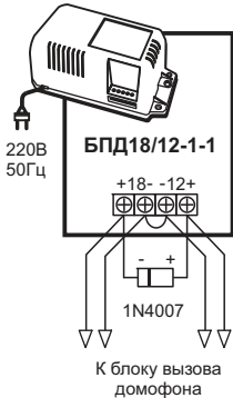
Рисунок 2 - Схема включения диода
