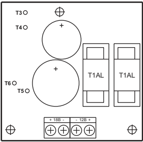
Рисунок 1 - Расположение элементов на плате блока питания БПД18/12-1-1
