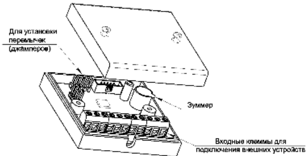
Рисунок 1 – Внешний вид и элементы подключения
