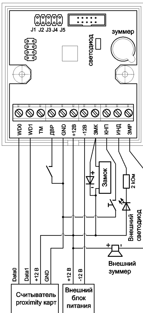
Рисунок 3 - Подключение СКУД со считывателем Wiegand
