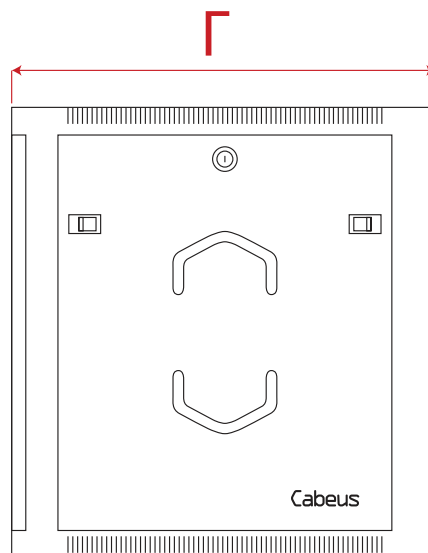
Вид сбоку
