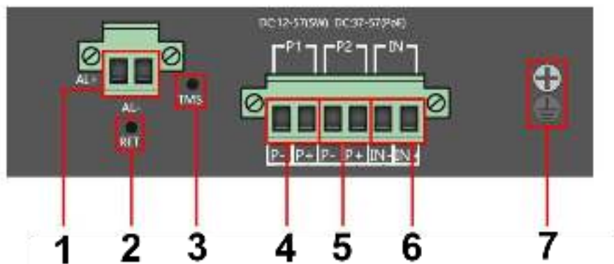
Рис. 3 Коммутатор SW-81602/ILS(port 90W, 600W), разъемы и кнопки на верхней панели
