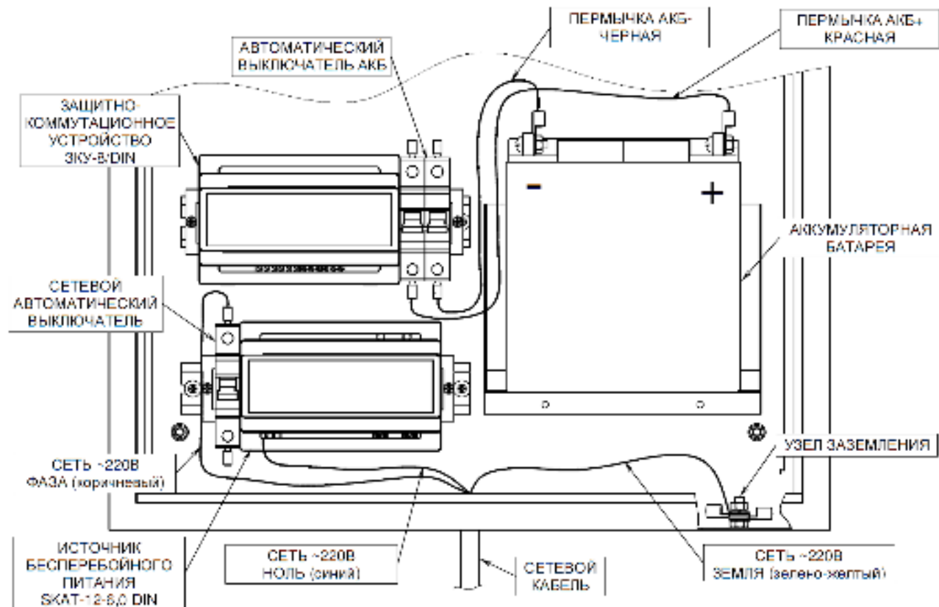
Рисунок 2 – подключение сетевого кабеля и АКБ
