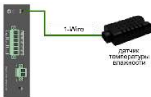
Рис.8 Схема подключения внешнего датчика температуры и влажности
