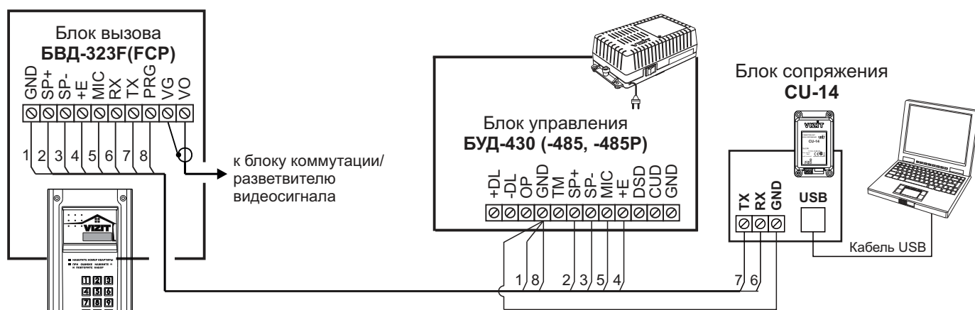
Рисунок 14 - Схема соединений блока сопряжения с блоками управления БУД-430 (-485, -485P)
