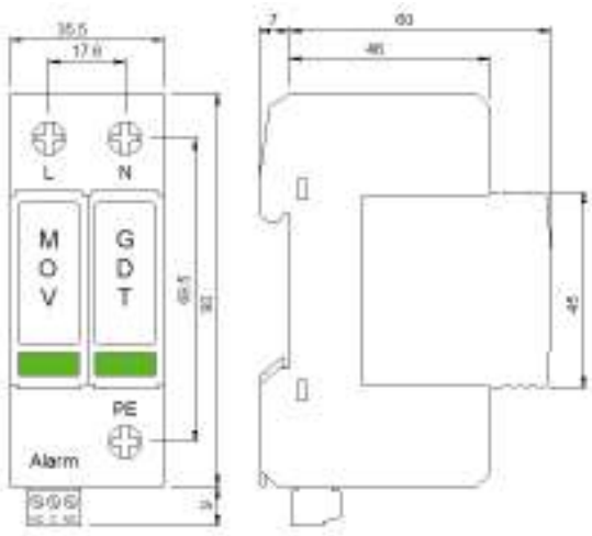
Рис. 1. Внешний вид и габариты TL240L385-1PN
