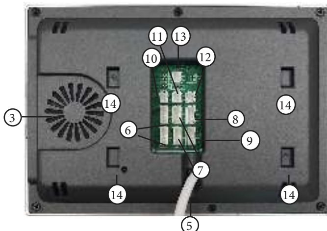
Конструкция монитора
