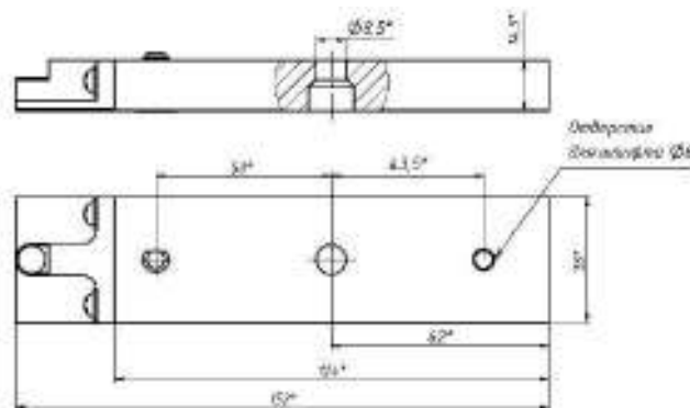
Рисунок 5- Габаритный чертеж якоря
