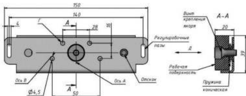
Рисунок 7- Якорная часть замка варианта «Н»
