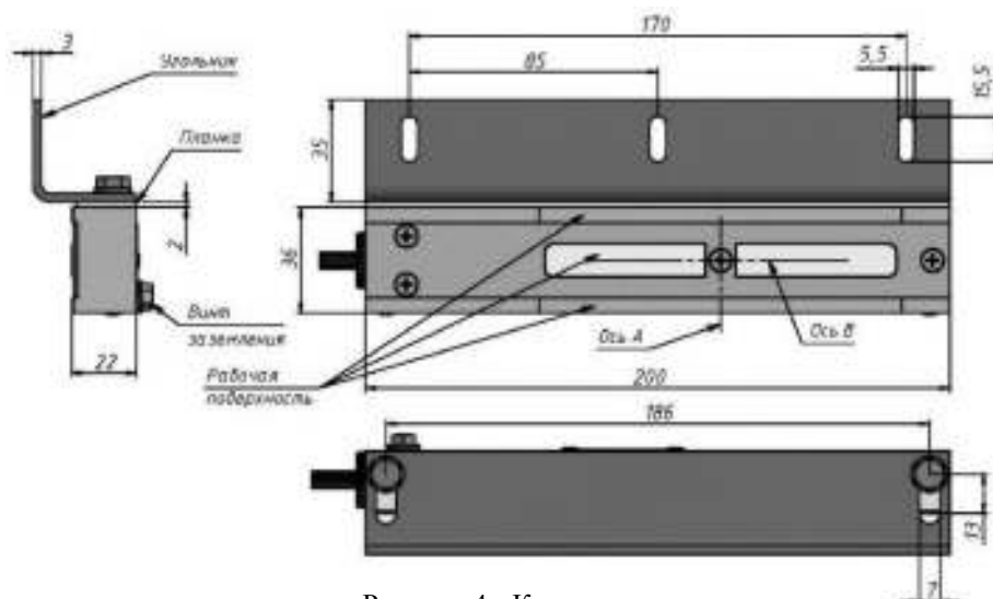
Рисунок 4 - Корпусная часть
