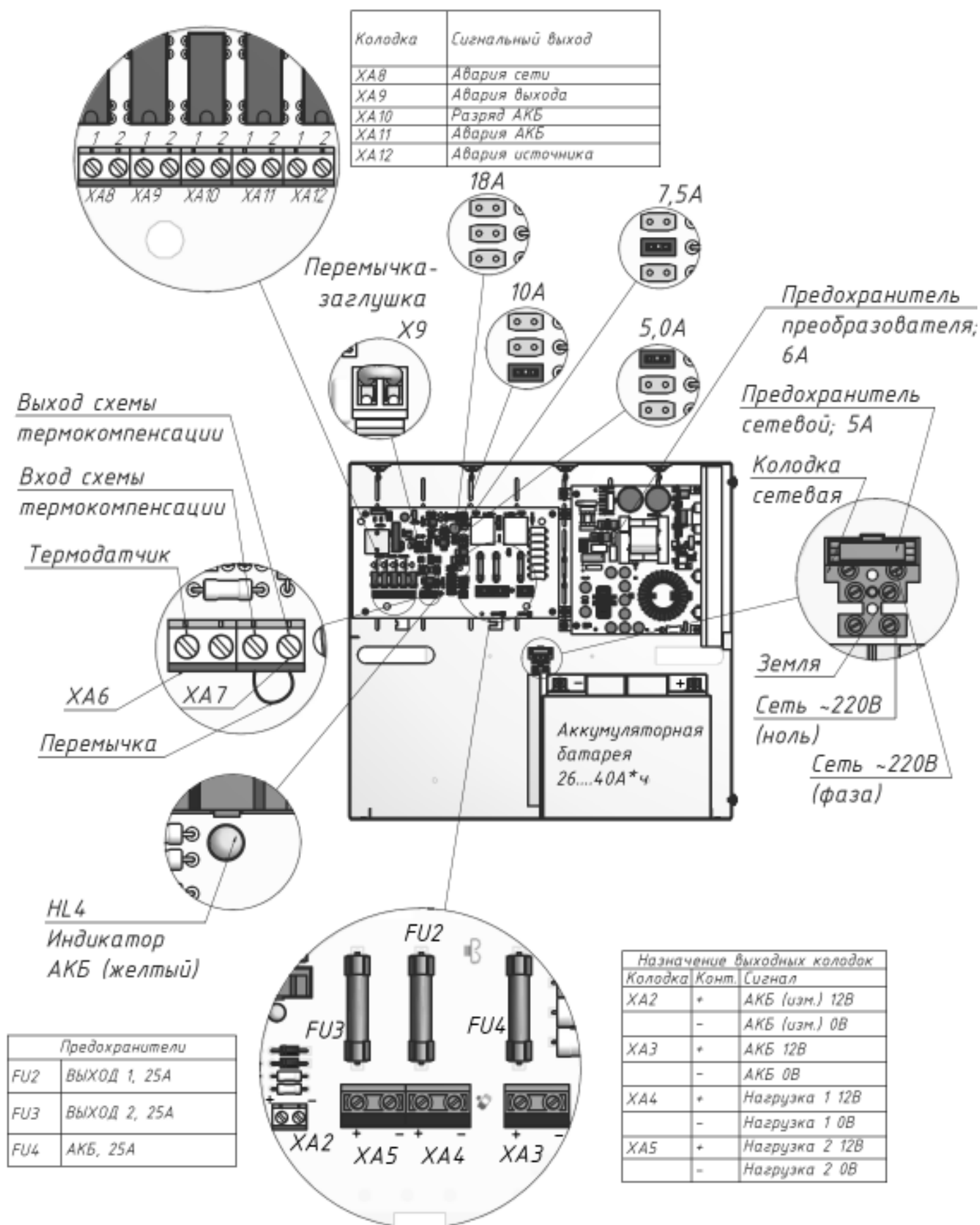
Рисунок 1 Общий вид источника с открытой крышкой
