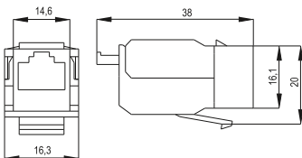
Рисунок/Figure 2 – CS1-1C5EU-12, CS1-1C06U-12
