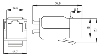
Рисунок/Figure 6 – CS1-1C5ES-T2, CS1-1C06S-T2, CS1-1C6AS-T2, CS1-1C06S-T2-D, CS1-1C6AS-T2-D
