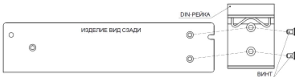
Рисунок 2 – крепление DIN-рейки.
