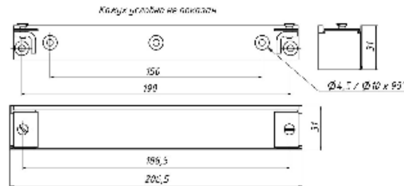
Рисунок 2 – Габаритно-установочные размеры кронштейна
