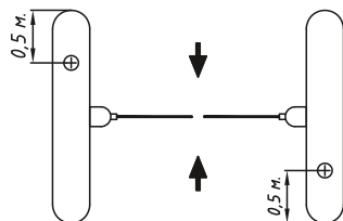
Рис. 7. Рекомендуемое размещение на турникете терминала R20-Face (8T) всех модификаций
