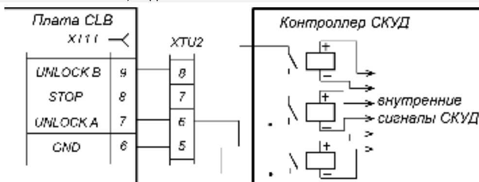
Рисунок 8. Управляющие элементы внешнего устройства – нормально разомкнутый контакт реле
