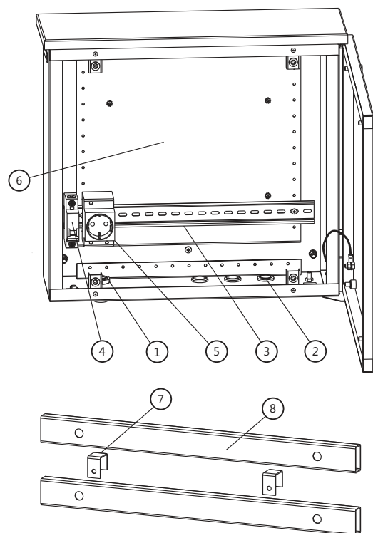
Рис.1 - Внешний вид и габаритные размеры бокса.
