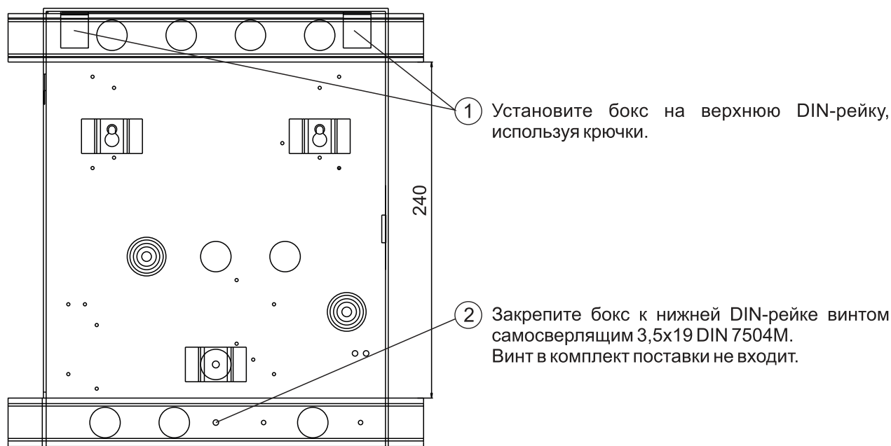
Рисунок 3 - Установка бокса на DIN-рейки
