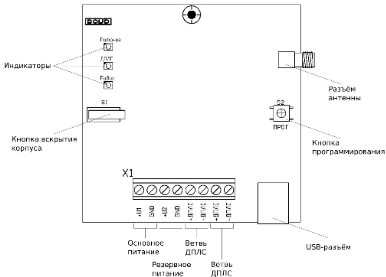
Рисунок 2.2 Расположение элементов на плате
