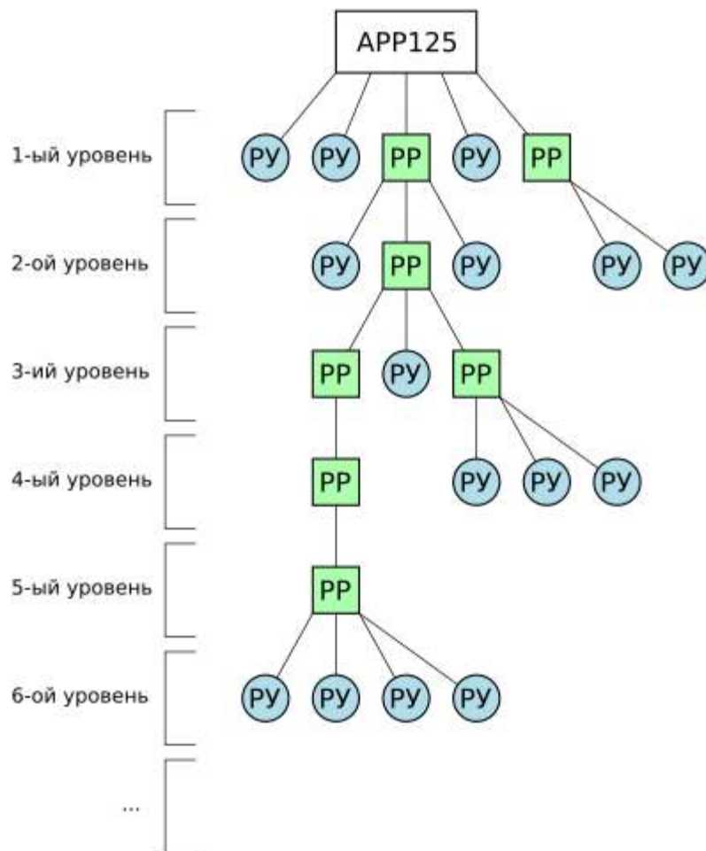
Рисунок 1.2 Цепь ретрансляции
