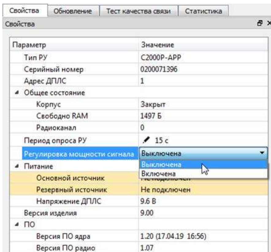
Рисунок 2.26 Управление мощностью сигнала
