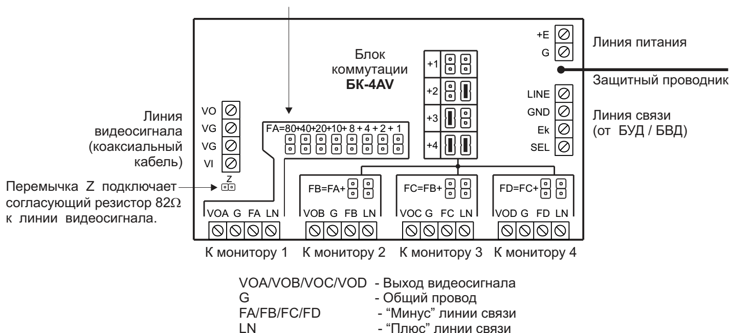
Рисунок 3 - Расположение клемм, назначение цепей и перемычек
