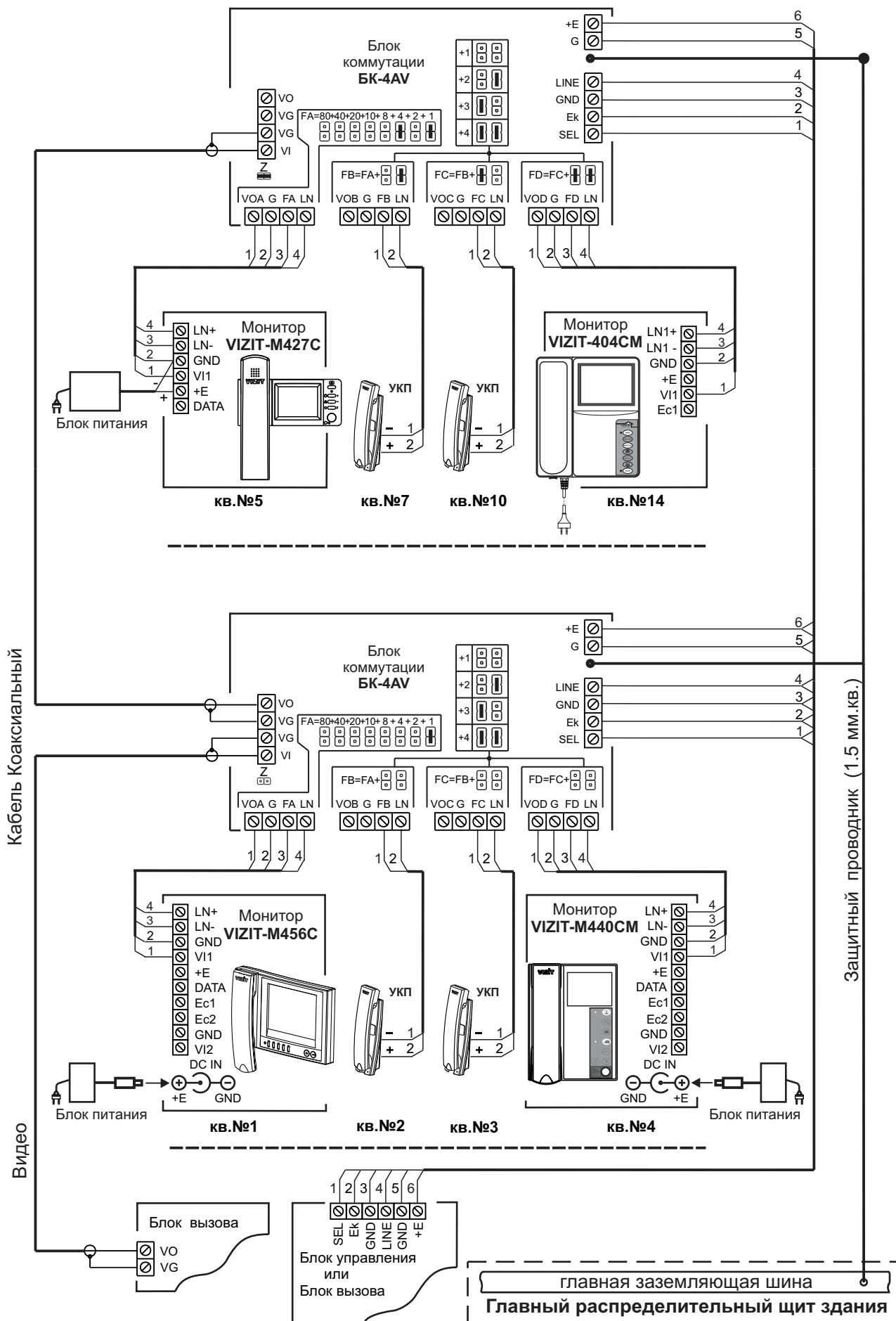
Рисунок 6 - Видеодомофон с применением блока коммутации БК-4AV
