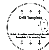
Рисунок 2-1 Шаблон крепления
