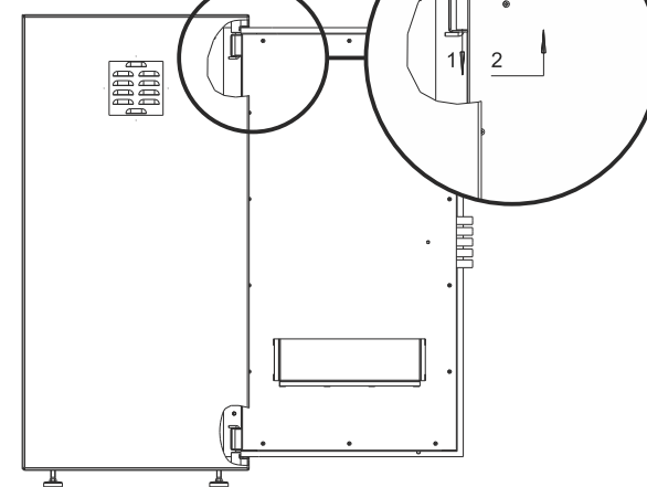
Снятие двери
