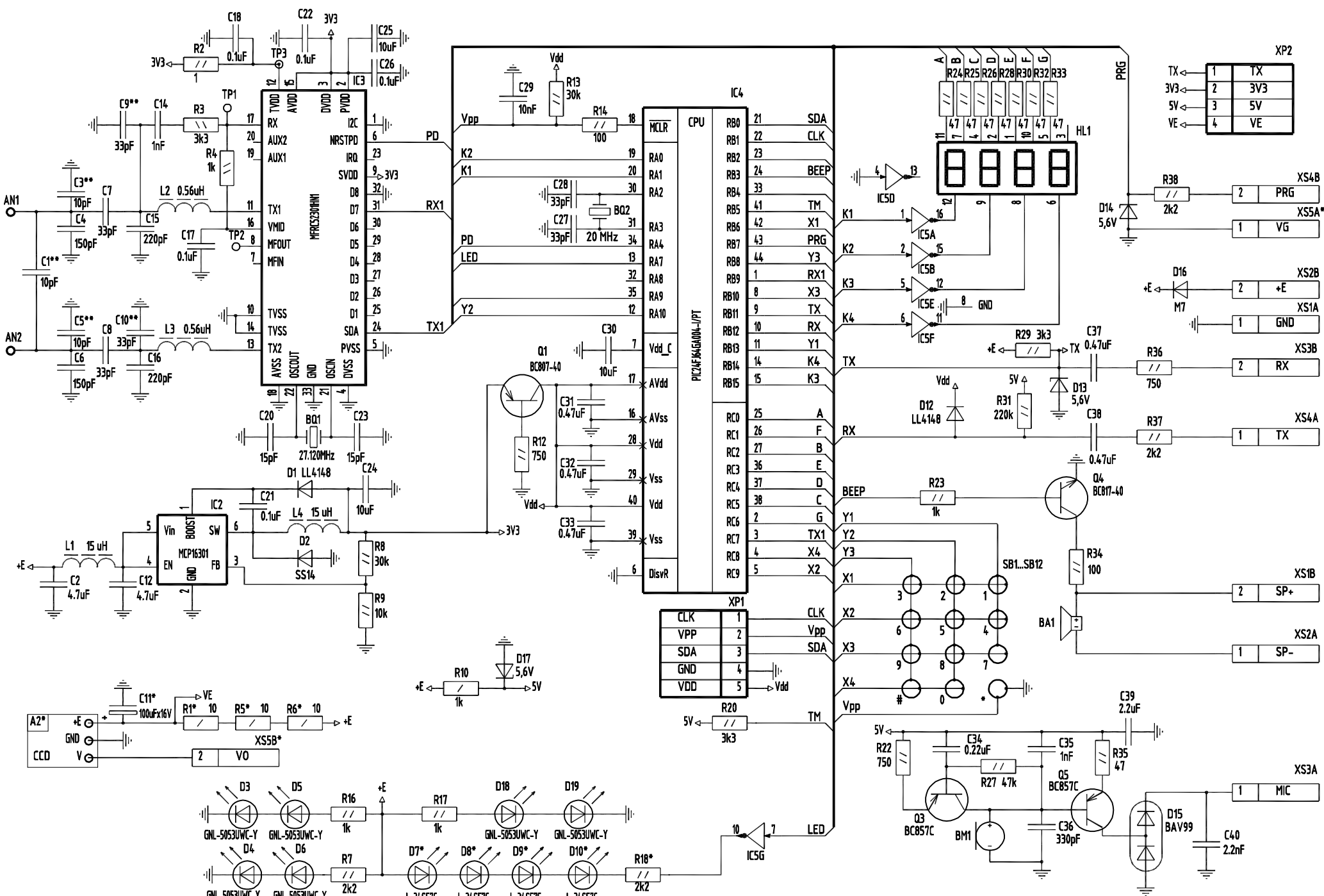
Блок вызова БВД-323FCP Схема электрическая принципиальная
