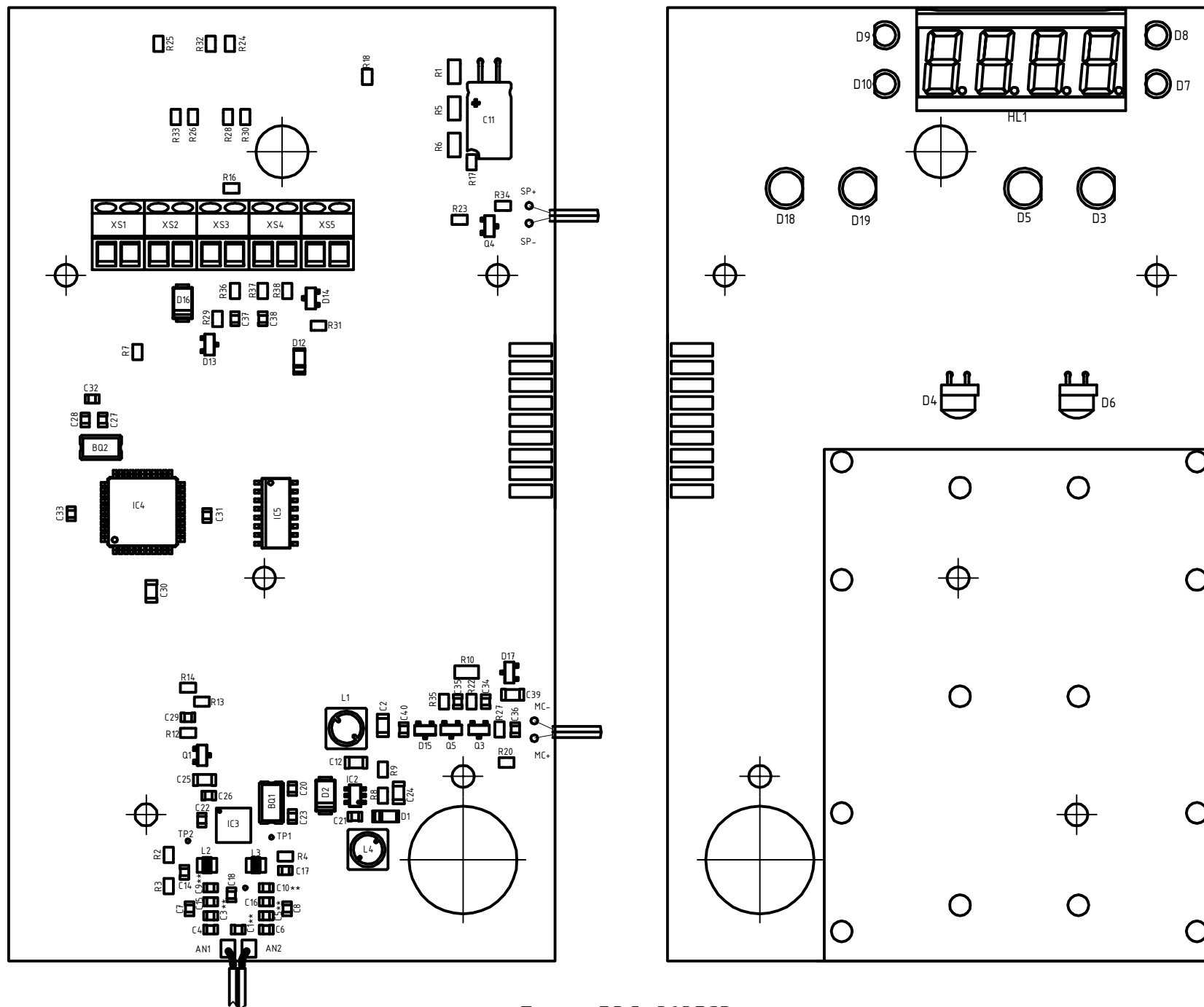
Плата БВД-323FCP Сборочный чертеж
