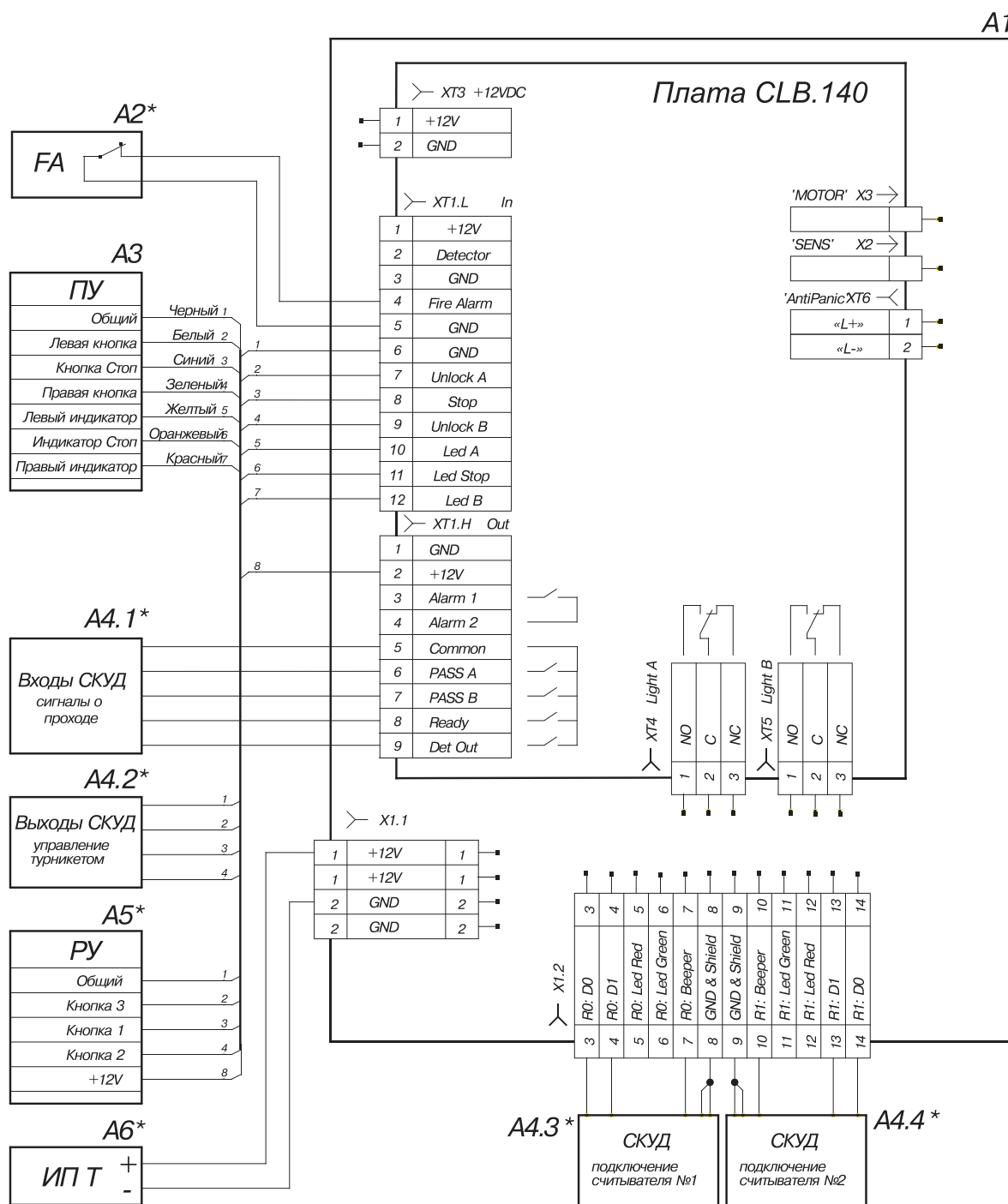
Схема соединений турникета PERCo-TB01.9A и дополнительного оборудования
