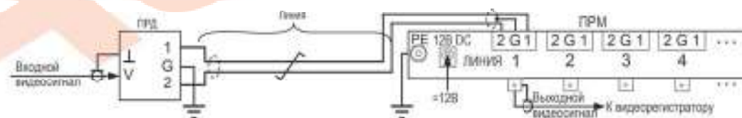
Рис.2 Схема включения комплекта АПВС-TVI (ПРД) и АПВС-К8-TVI (ПРМ)
