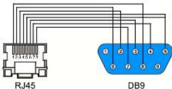
Рис.2 Распиновка разъемов кабеля Console-RJ45-DB9F
