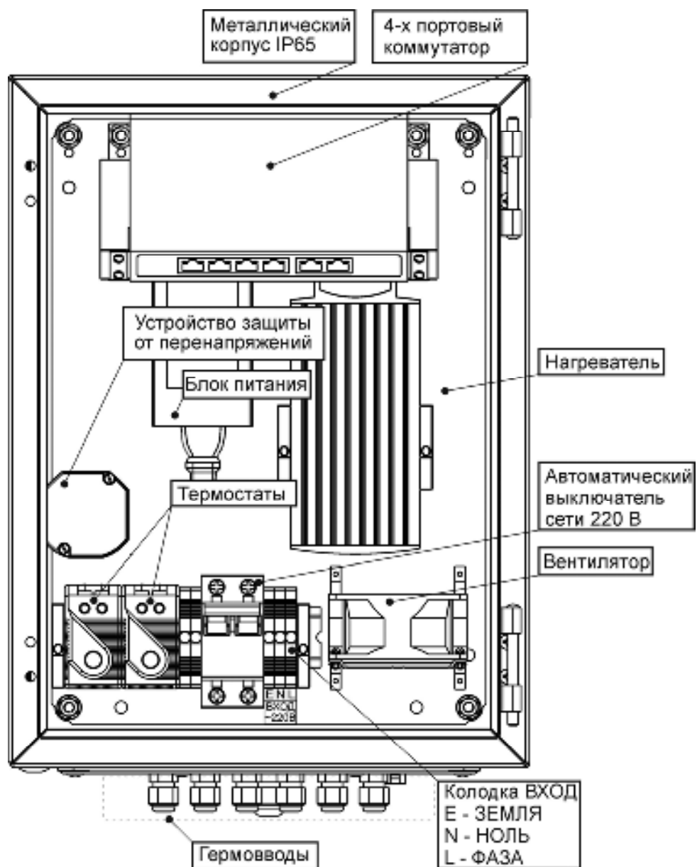
Рисунок 3 - вид изделия с открытой дверцей
