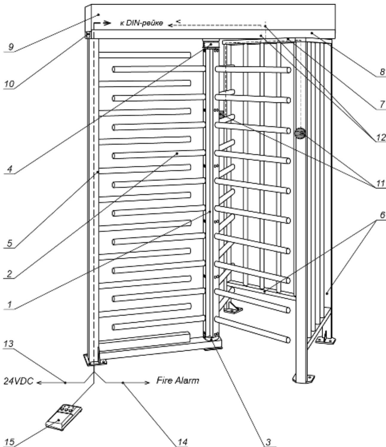
Рисунок 2. Устройство турникета:
