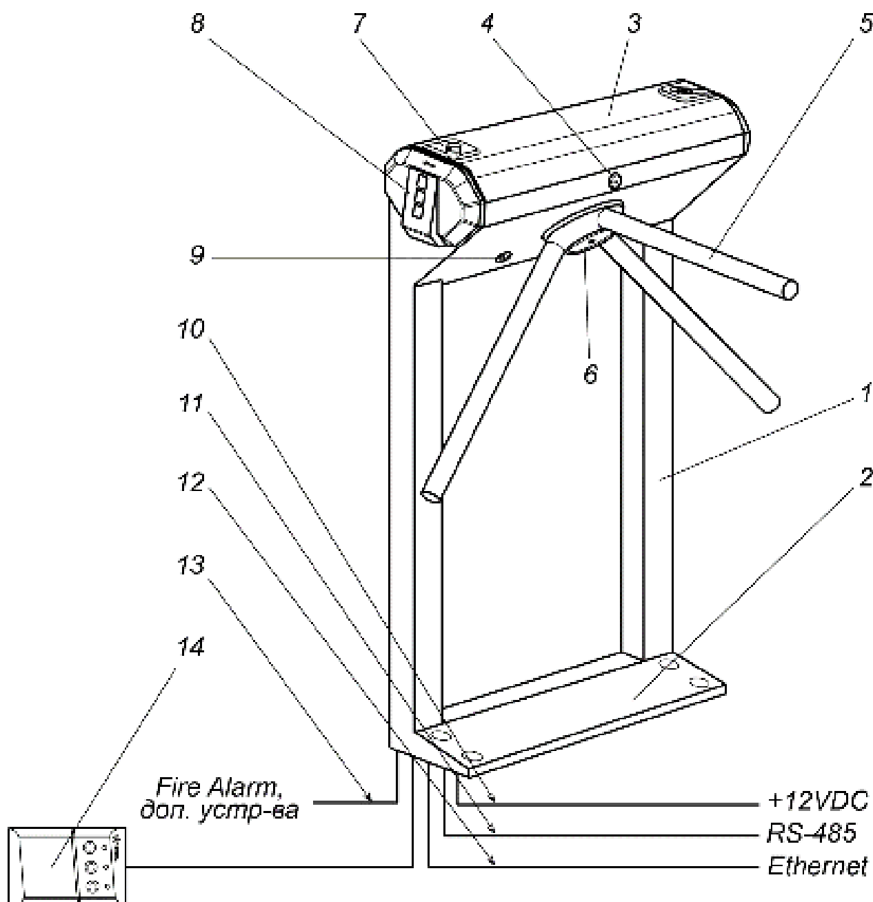
Рисунок 2. Устройство ЭП
