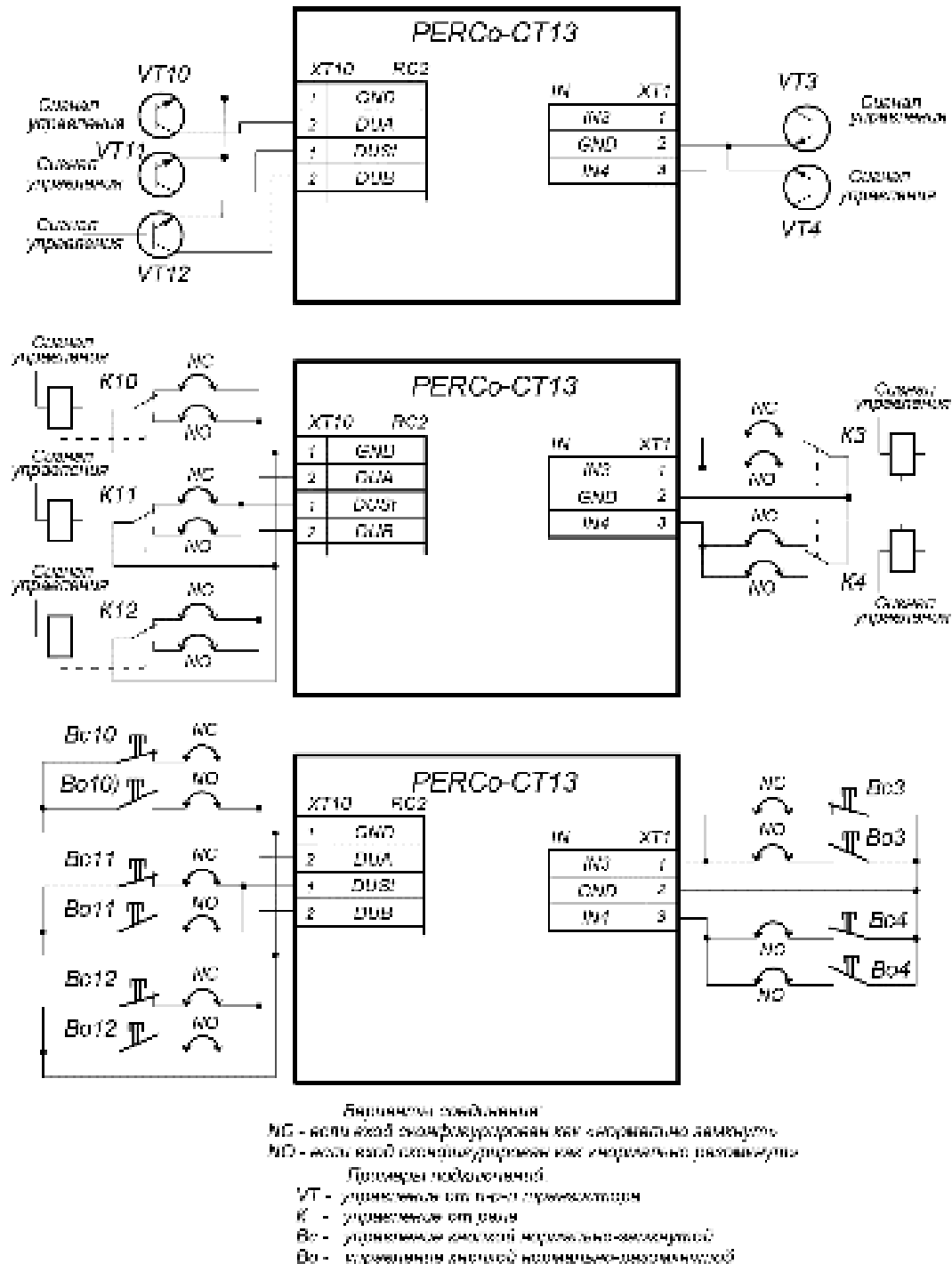
Рисунок 24. Схема подключений доп. оборудования к входам контроллера
