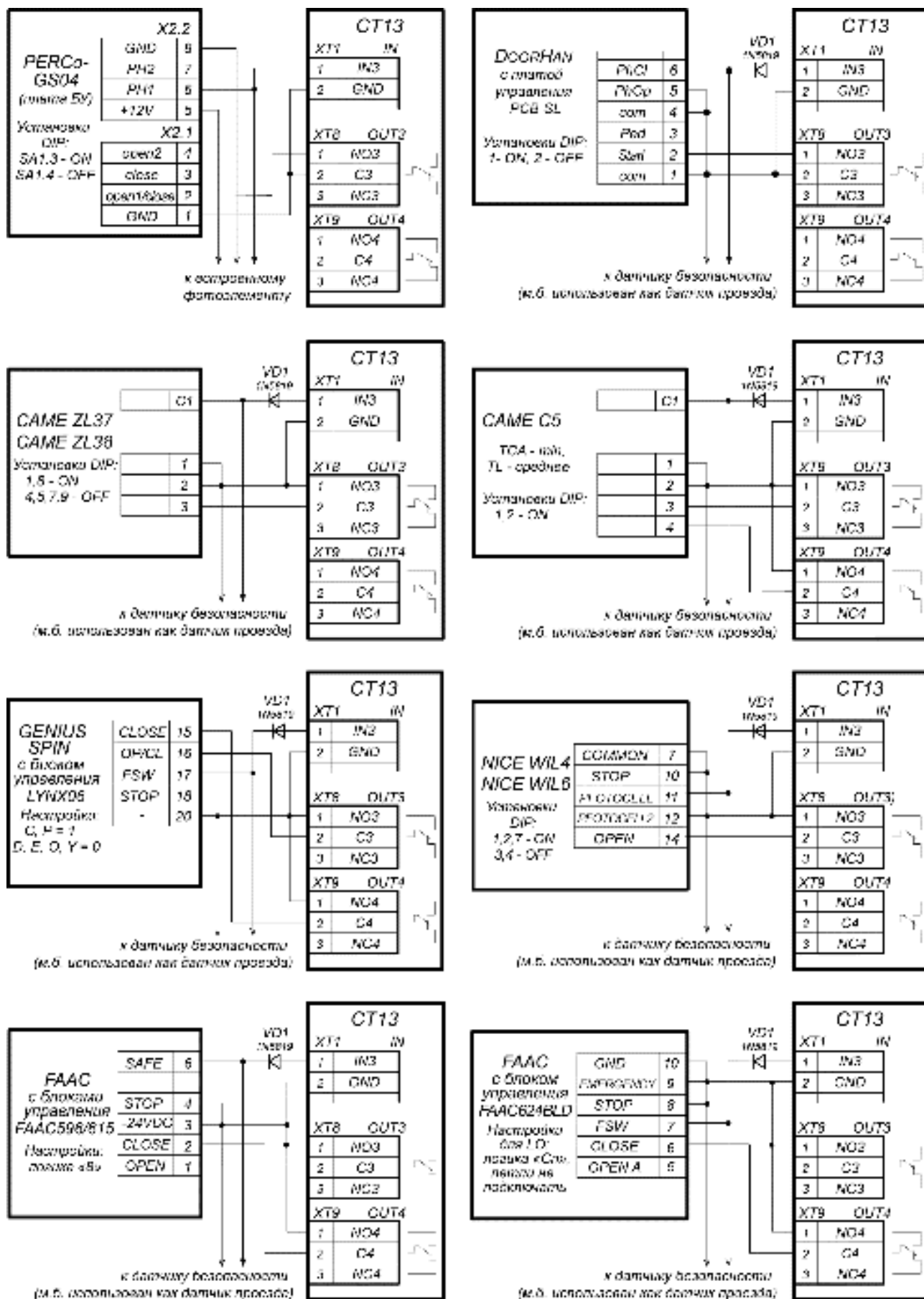
Рисунок 19. Примеры схем подключения шлагбаумов к контроллеру АТП
