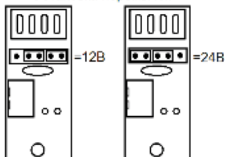
Установка перемычек
