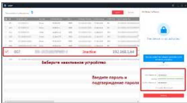
Рисунок 3-4 SADP интерфейс
