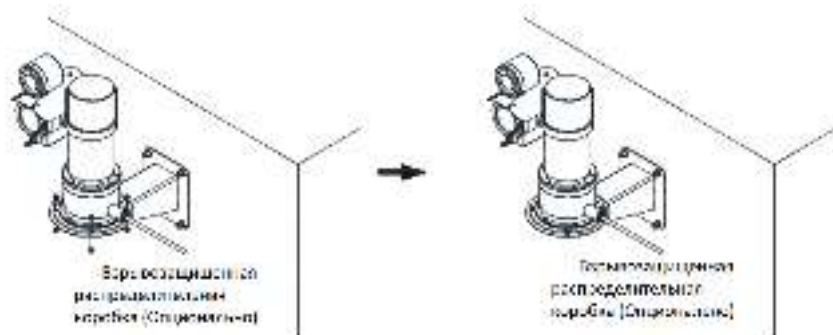
Рисунок 2-4 Крепление системы позиционирования
