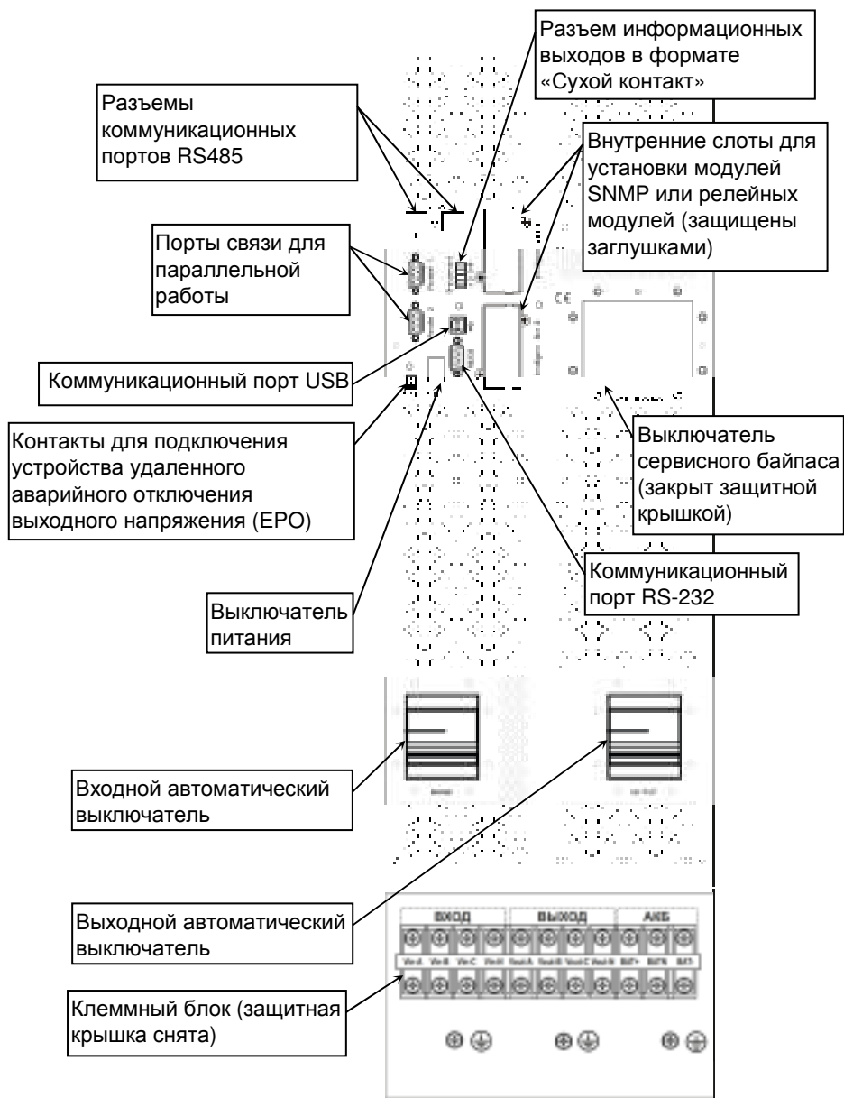
Рисунок 2 — Общий вид задней панели изделия со снятой крышкой клеммного блока
