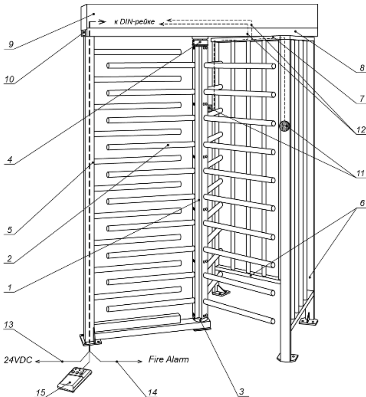
Рисунок 2. Устройство турникета:
