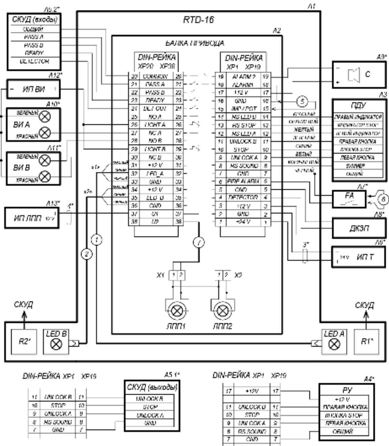
Рисунок 21. Схема подключения турникета и дополнительного оборудования 1
