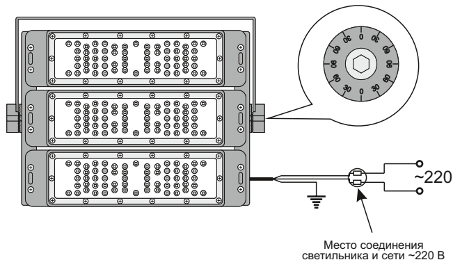
Рисунок 2 — Схема подключения изделия
