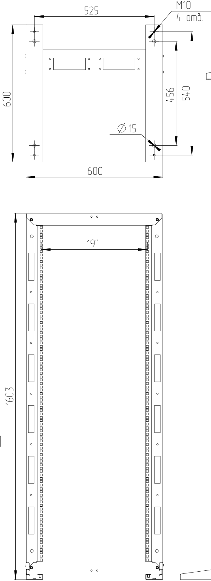
Стойка СТК-33U
