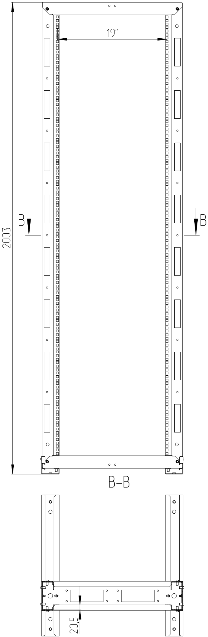
Стойка СТК-42U
