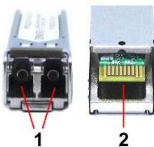
Рис.2 SFP модули SFP-M2LC15-G-850-850, SFP-M2LC15-G-850-850-I, разъемы спереди/сзади
