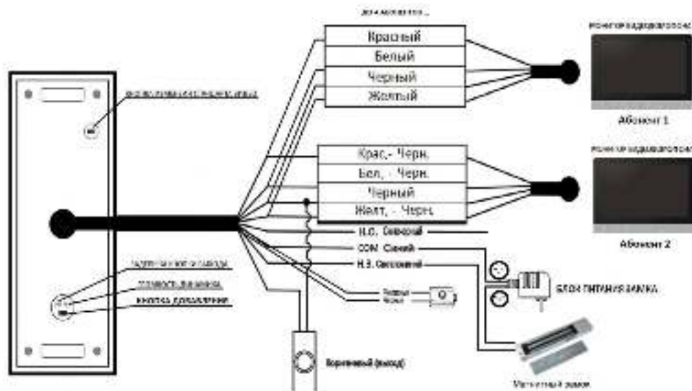
Рисунок 1. Подключение
