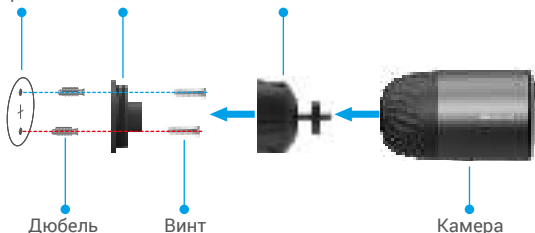
Рисунок 2. Монтаж с помощью резьбового основания
