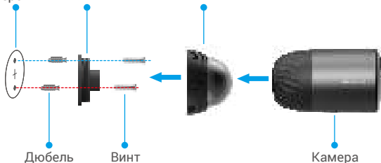
Рисунок 1. Монтаж с помощью магнитного основания
