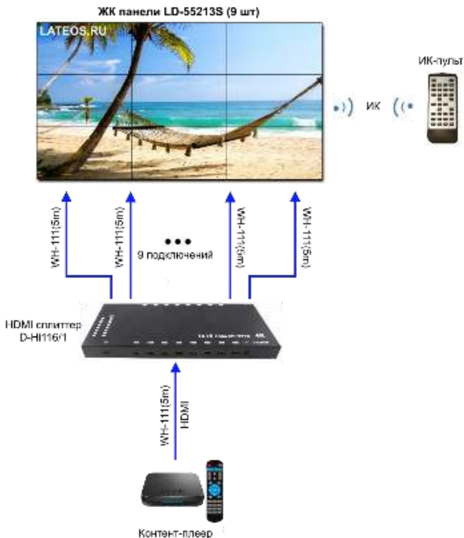
Рис.1 Схема подключения типового комплекта VW3355W
