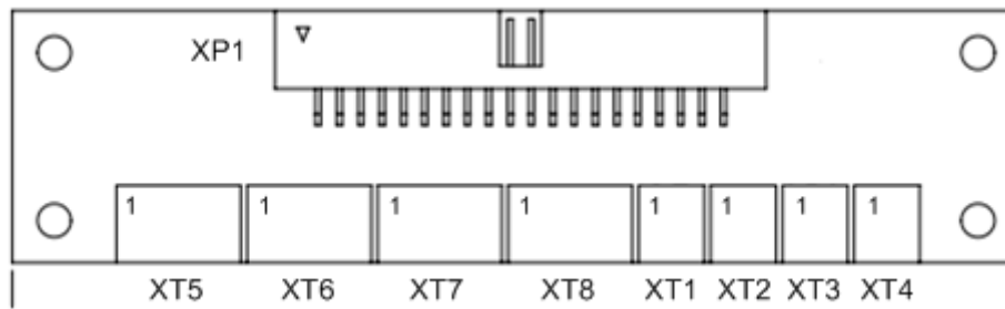
Рис. 12.2 Клеммные колодки XT1 – XT8
