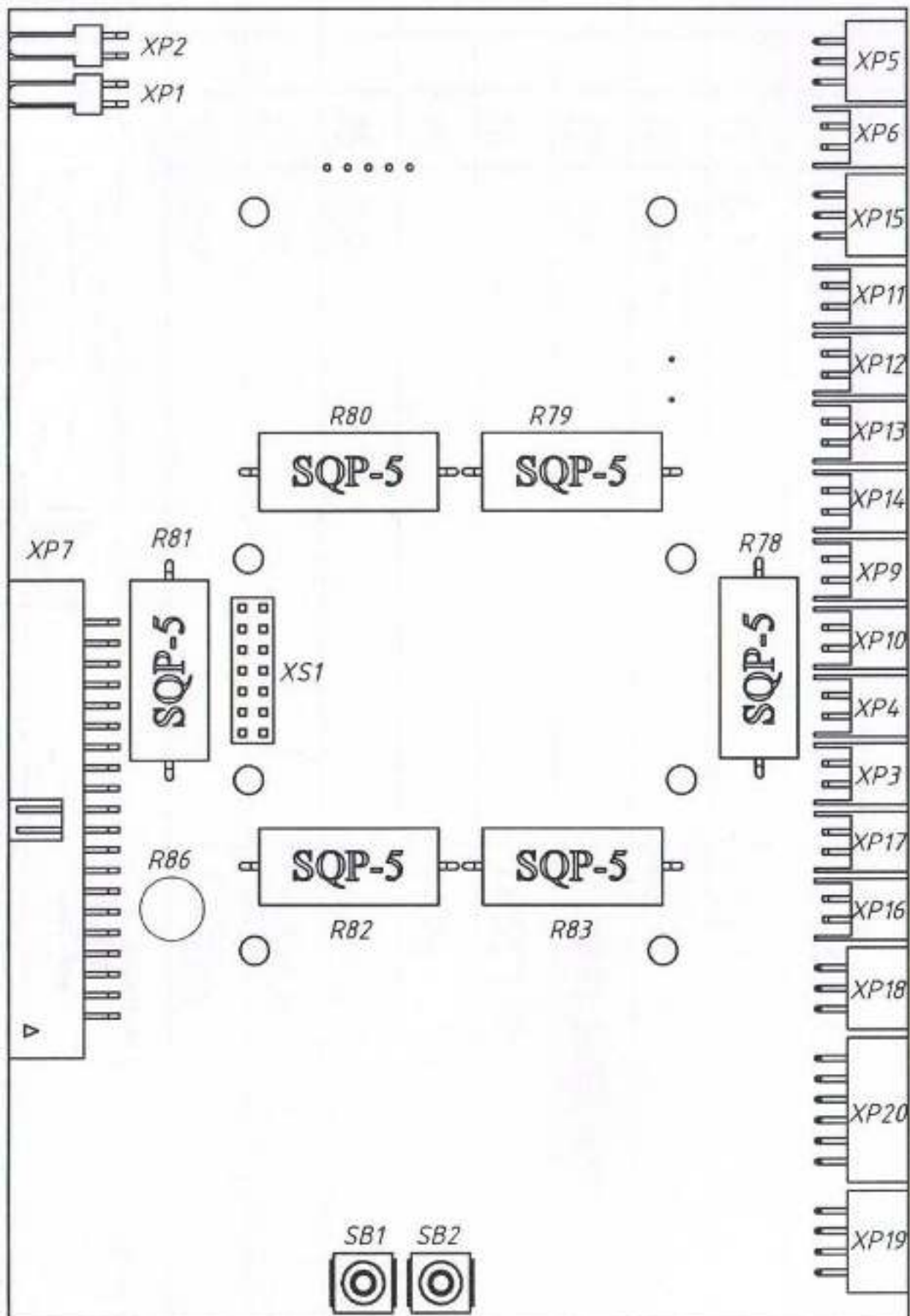
Рис. 12.1. Плата управления
