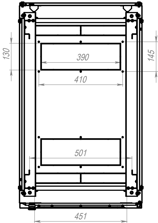
A-A
