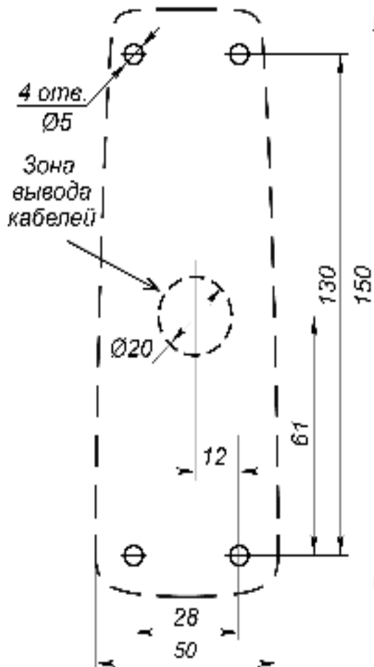
Рисунок 2. Разметка отверстий для установки контроллера (пунктиром показаны габариты корпуса контроллера)
