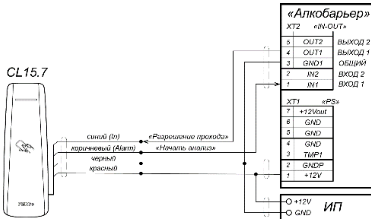
Рисунок 10. Схема подключения ВВУ на примере алкотестера
