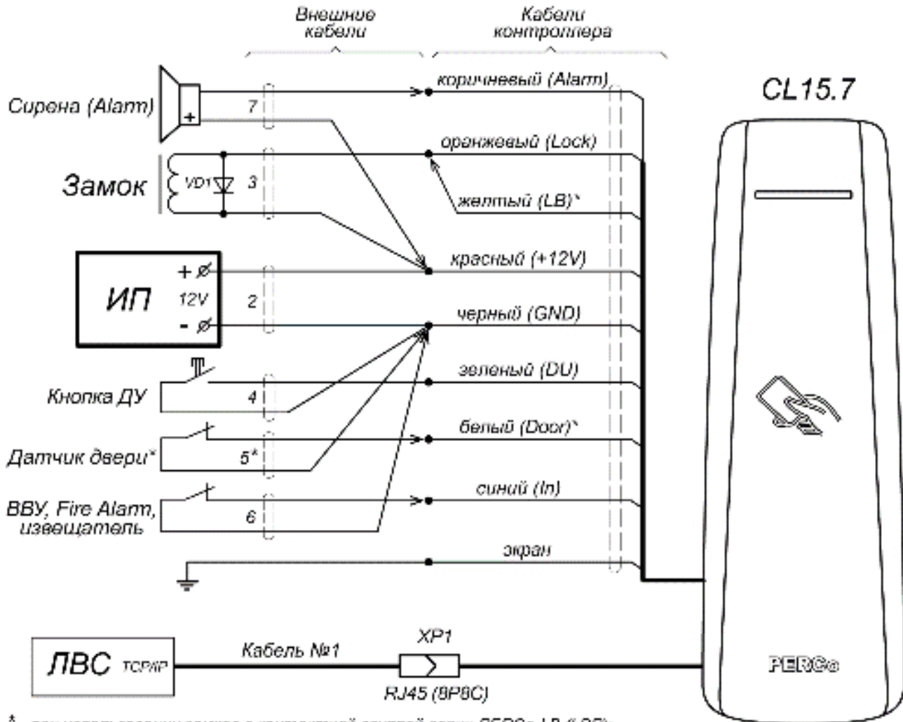
Рисунок 3. Схема подключений контроллера для управления односторонним замком
