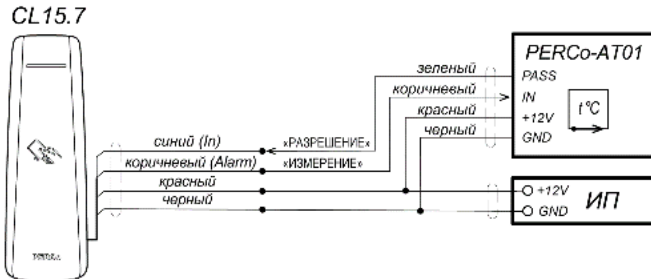
Рисунок 12. Схема подключения пирометра PERCo-AT01 к контроллеру CL15.7
