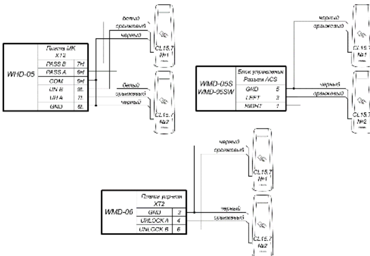
Рисунок 8. Схемы подключений калиток
