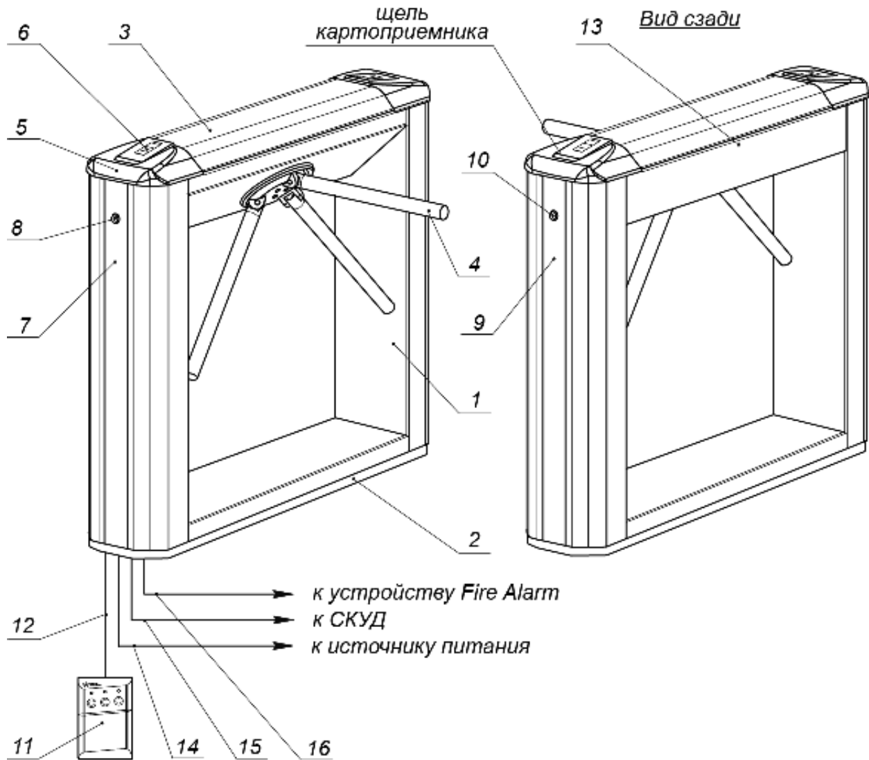
Рисунок 2. Устройство турникета
