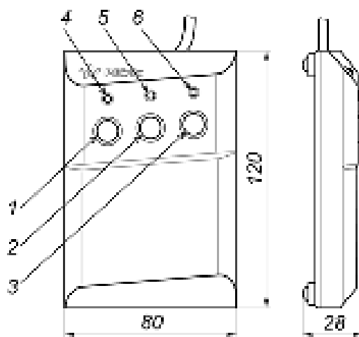
Рисунок 3. Общий вид и габаритные размеры ПДУ
