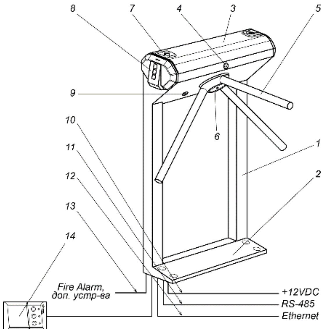
Рисунок 1. Устройство ЭП
