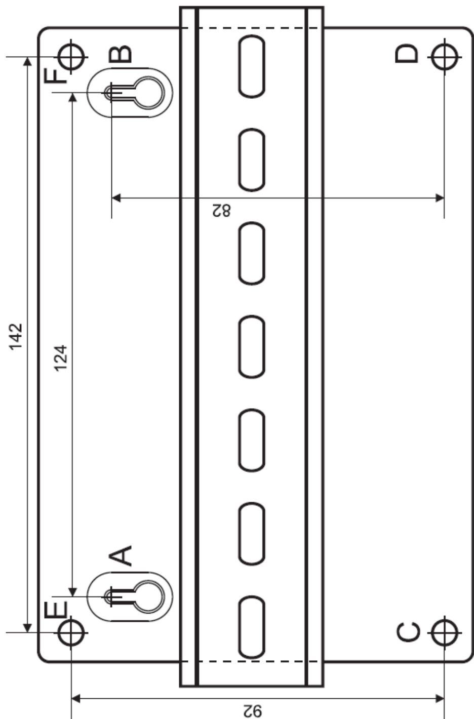
Рисунок 16. Шаблон для монтажа
