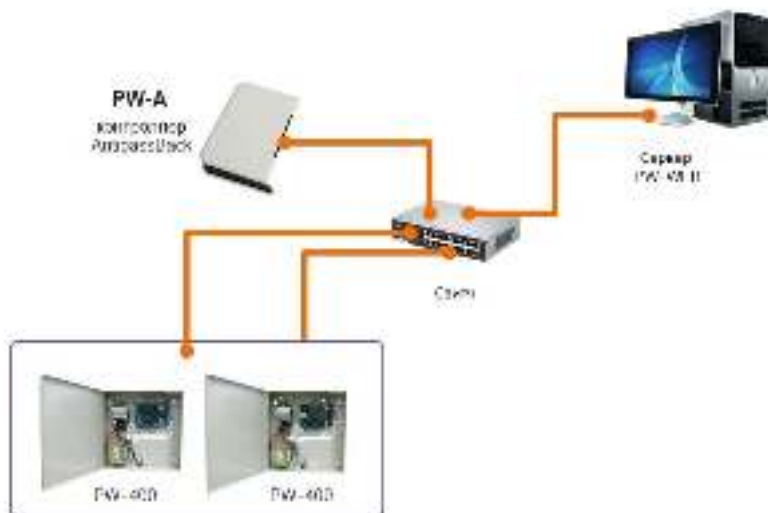
Рис 3. Пример локальной сети смешанного типа (Ethernet и Wi-Fi)
