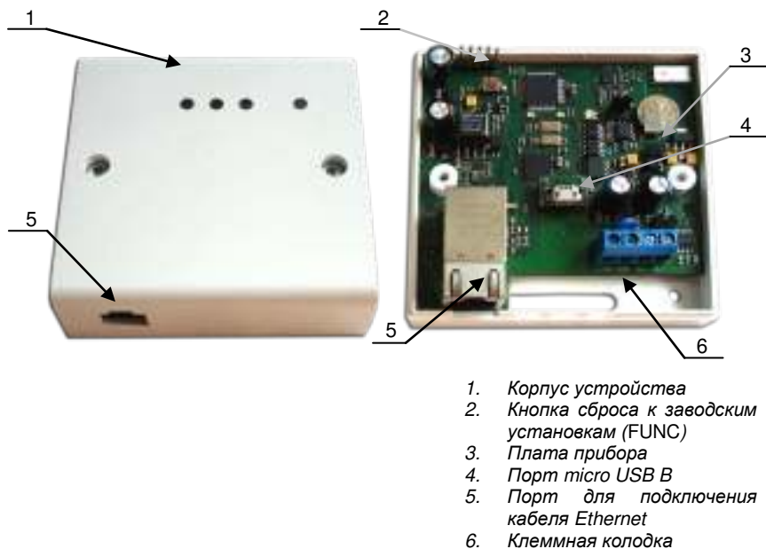
Рис. 1а. Внешний вид ProxWay PW-A модификации 1
