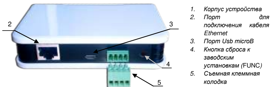
Рис. 1. Внешний вид ProxWay PW-A модификации 2
